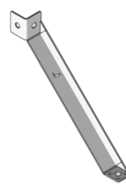
Укосина EFK 500
