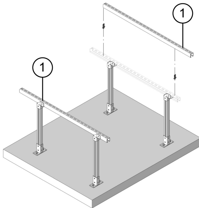
Рис. 13 1-Профиль EF.
