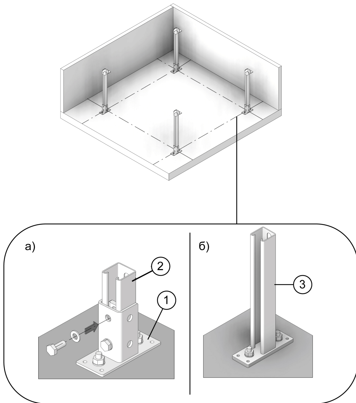
Рис. 5 Установка стойки
